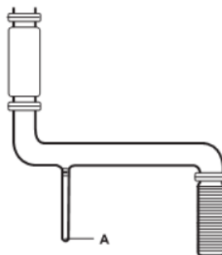
Сборник конденсата Длина ≈ 30мм (1.2") Диаметр ≈ 25.4мм (1") А - кран или пробка
